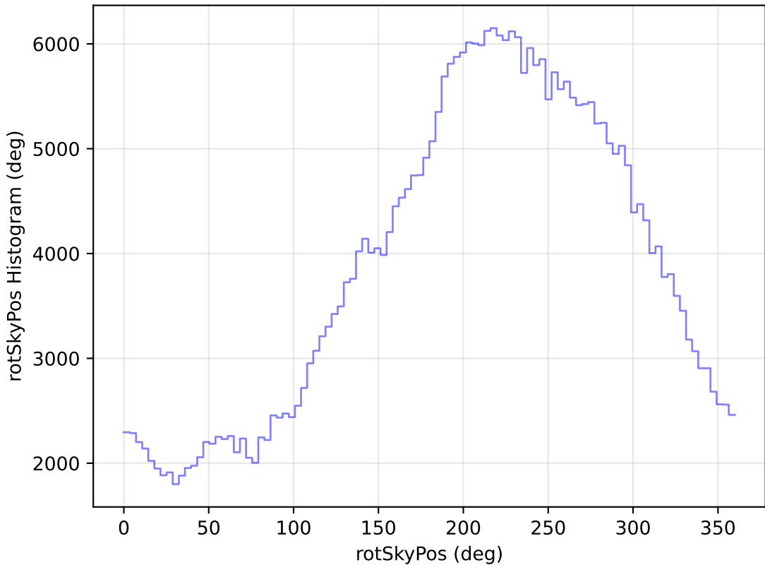
too_elab_r64_d3_ugrizy_v3.4_10yrs WFD y band: rotSkyPos Histogram
