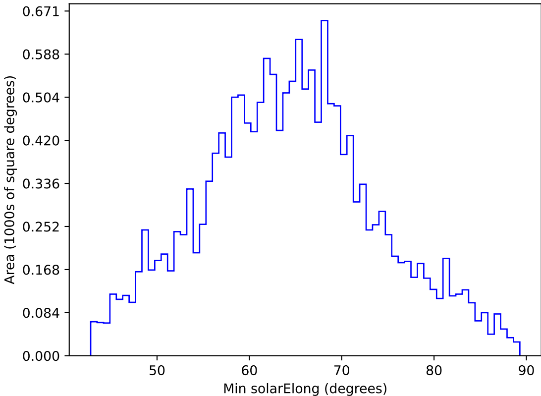
too_elab_r64_d3_ugrizy_v3.4_10yrs WFD y band: Min solarElong
