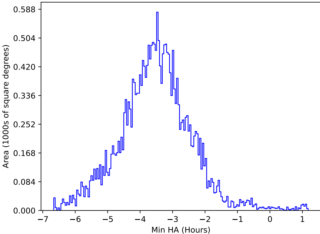
too_elab_r64_d3_ugrizy_v3.4_10yrs All sky y band: Min HA
