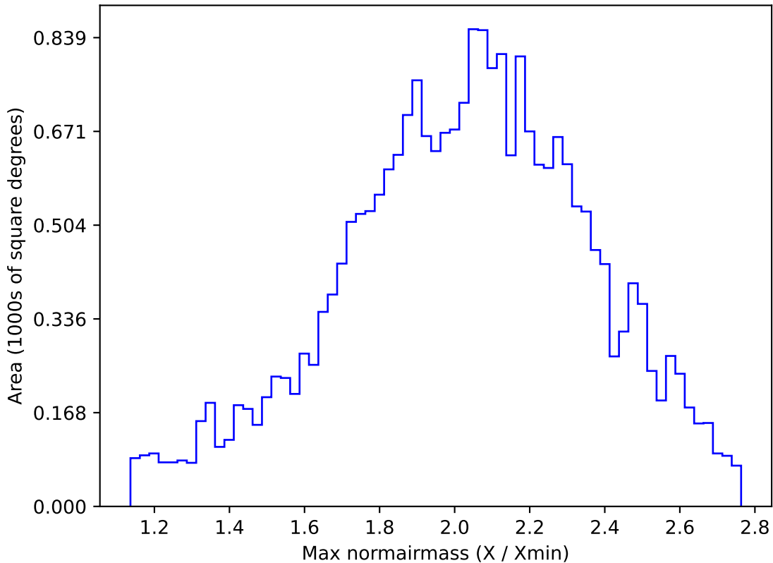
too_elab_r64_d3_ugrizy_v3.4_10yrs All sky y band: Max normairmass
