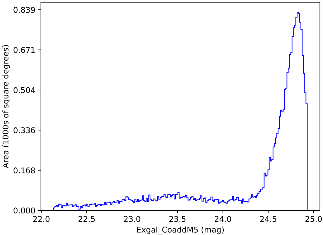
too_elab_r64_d3_ugrizy_v3.4_10yrs All sky y band: Exgal_CoaddM5
