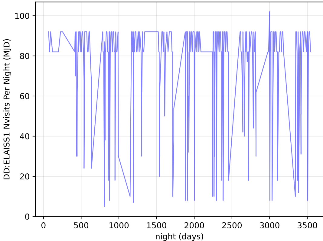
too_elab_r64_d3_ugrizyv3.4_10yrs all bands: DD:ELAISS1 Nvisits Per Night
