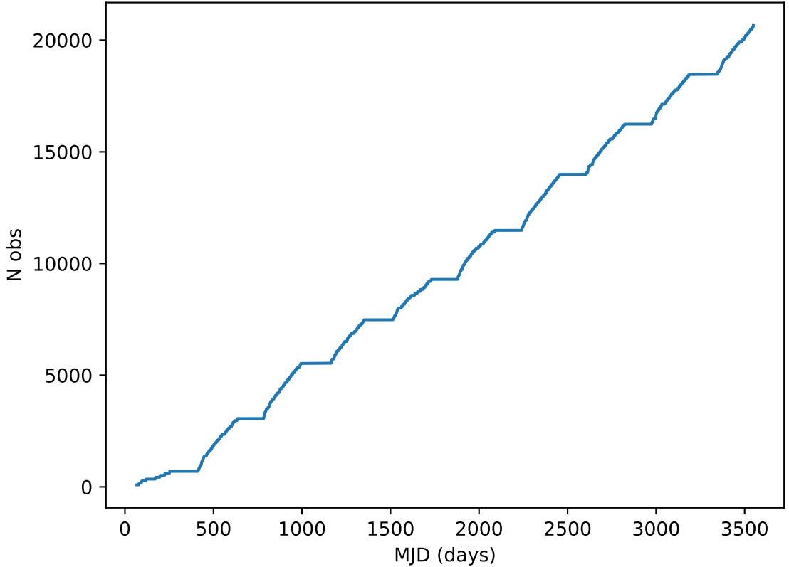
too_elab_r64_d3_ugrizy_v3.4_10yrs all bands: DD:ELAISS1 Cumulative NVisits
