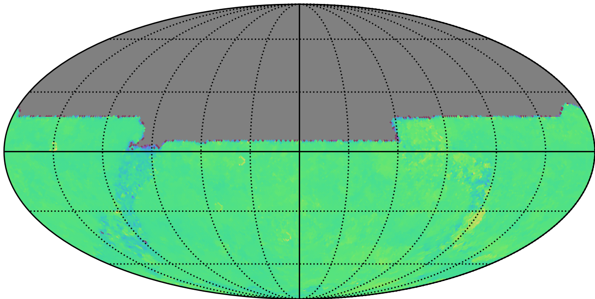
too_elab_r64_d3_gz_v3.4_10yrs u: Kuiper rotTelPos
