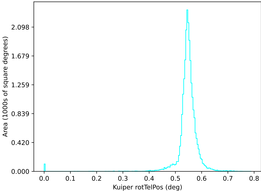
too_elab_r64_d3_gz_v3.4_10yrs u: Kuiper rotTelPos
