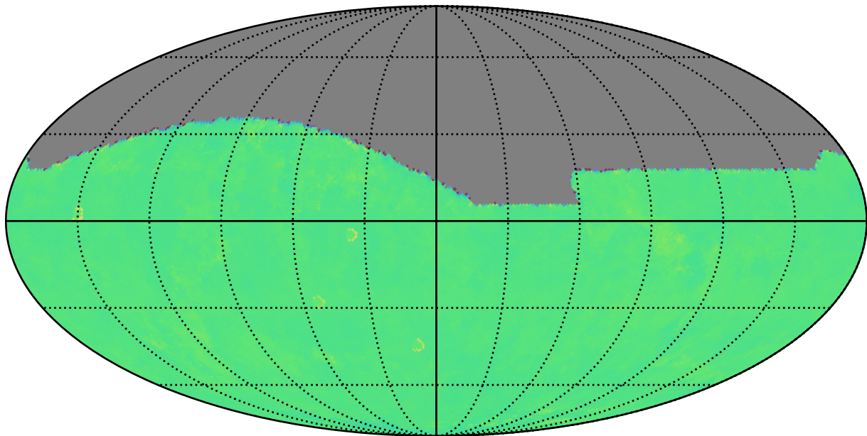
too_elab_r64_d3_gz_v3.4_10yrs i: Kuiper rotTelPos
