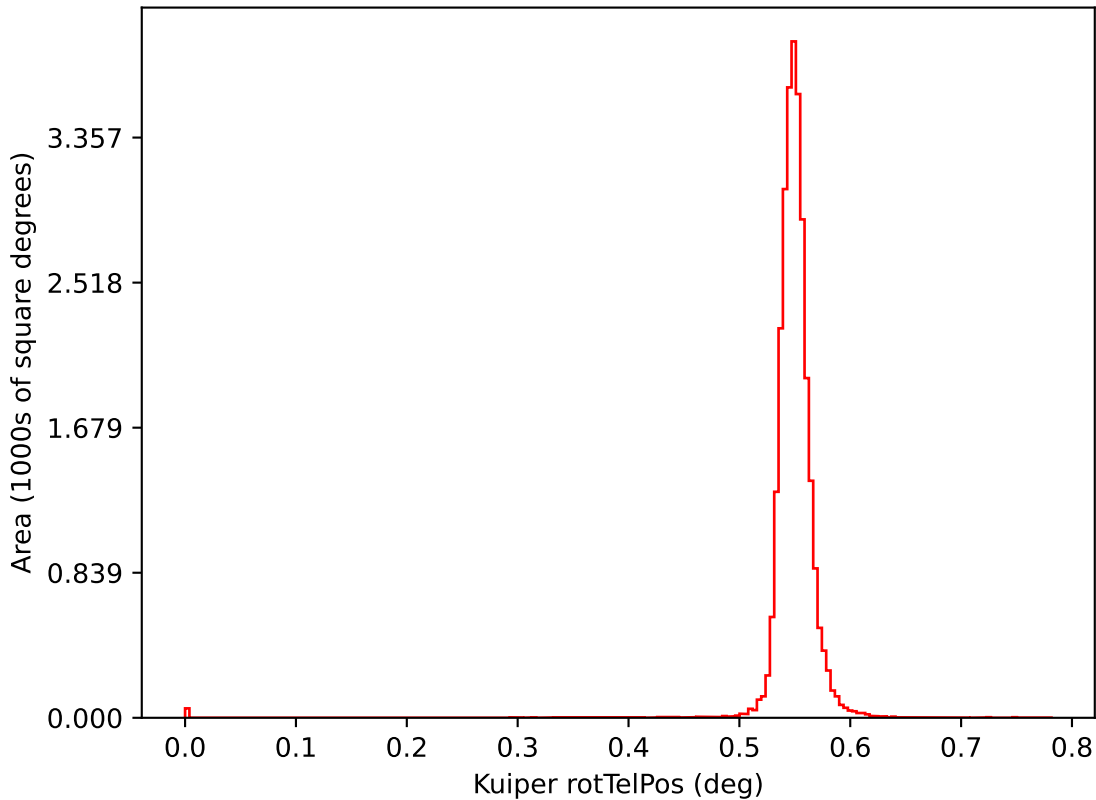
too_elab_r64_d3_gz_v3.4_10yrs i: Kuiper rotTelPos
