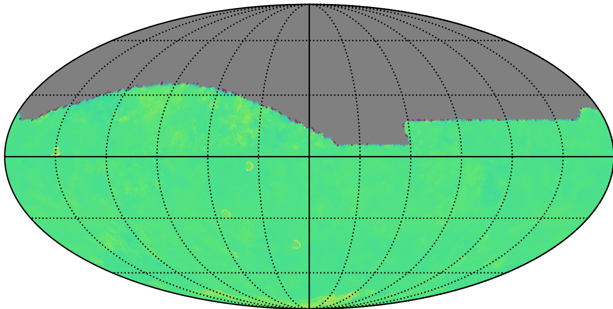
too_elab_r64_d3_griz_v3.4_10yrs z: Kuiper rotTelPos
