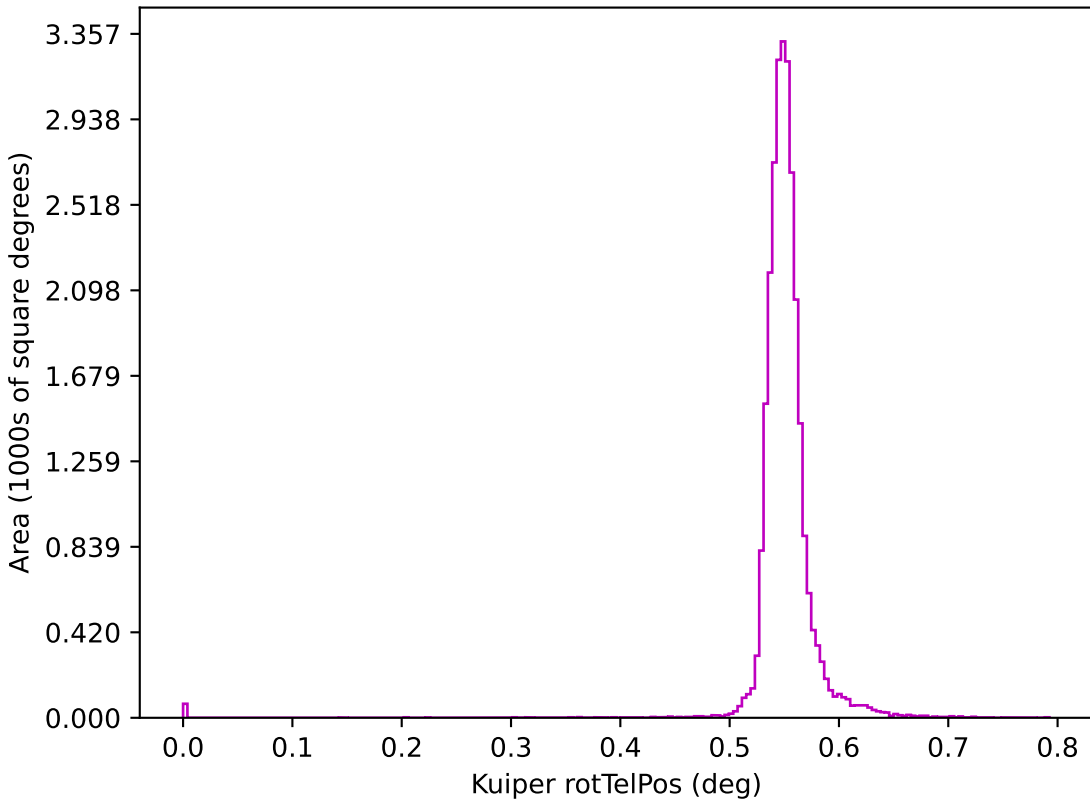
too_elab_r64_d3_griz_v3.4_10yrs z: Kuiper rotTelPos
