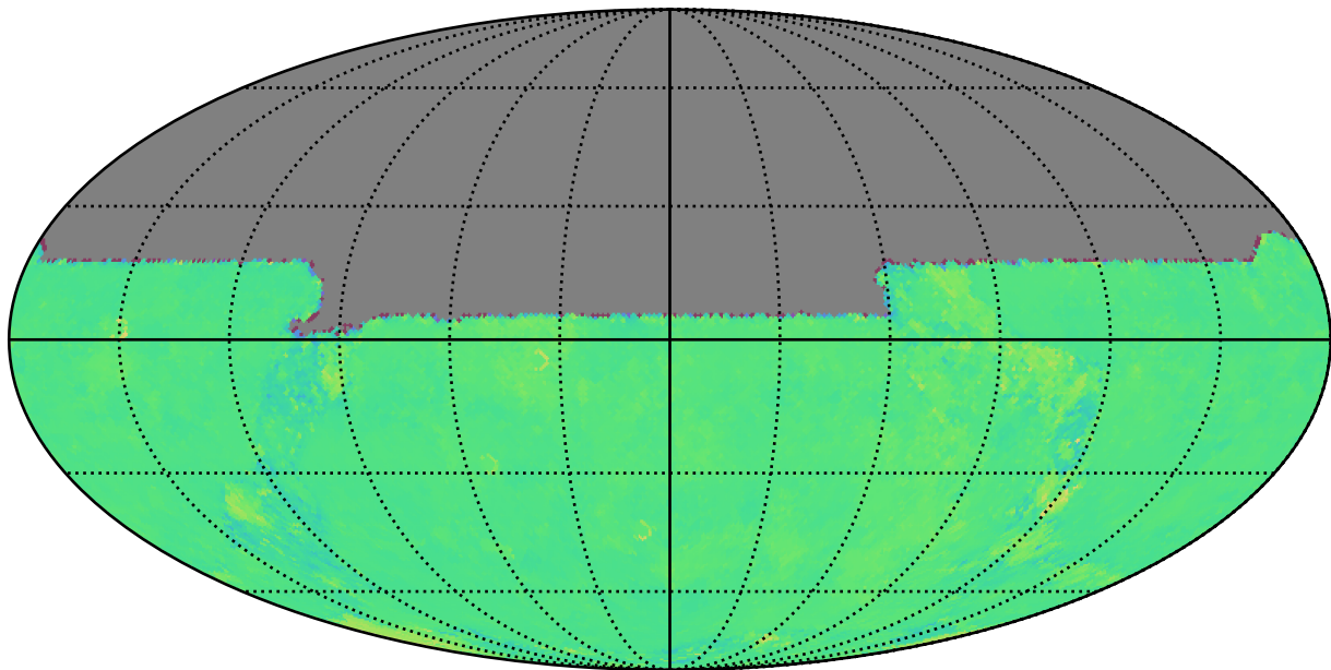
too_elab_r64_d3_griz_v3.4_10yrs u: Kuiper rotTelPos
