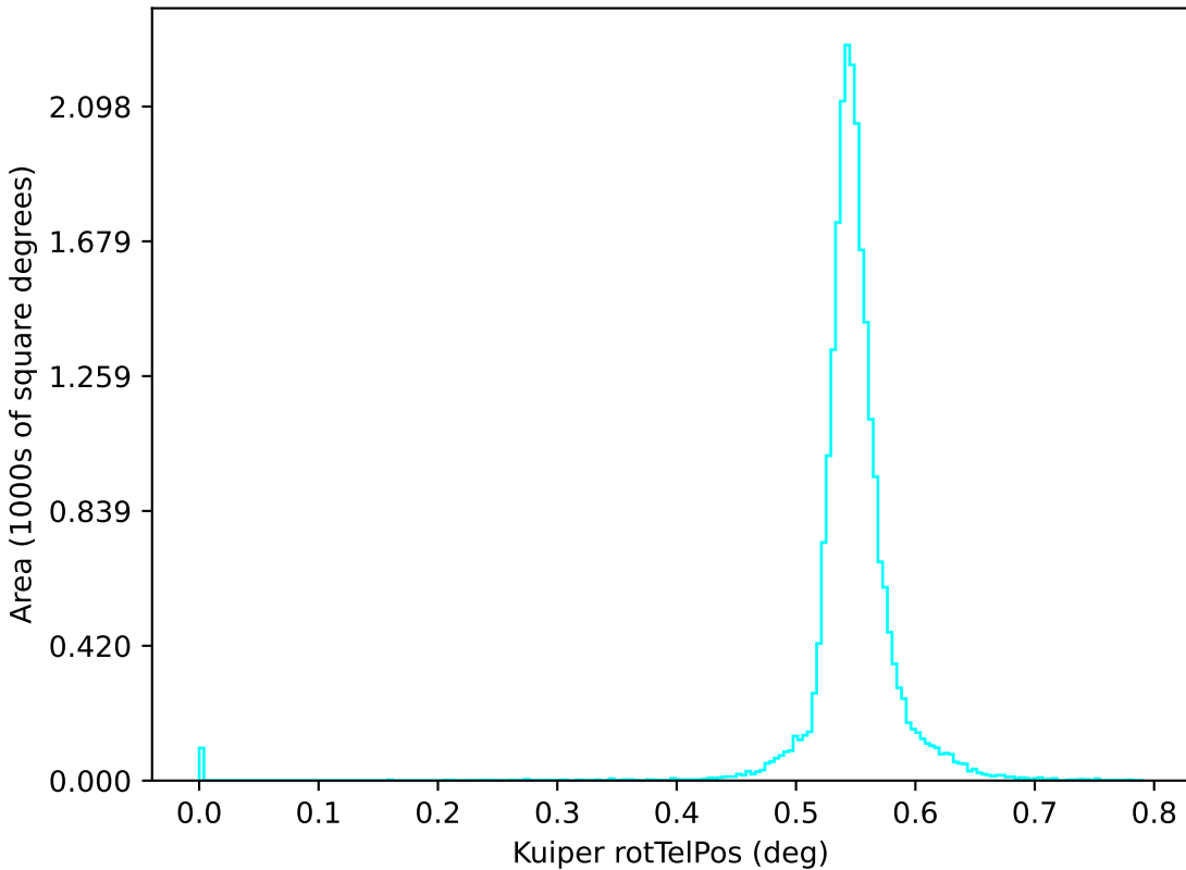
too_elab_r64_d3_giz_v3.4_10yrs u: Kuiper rotTelPos
