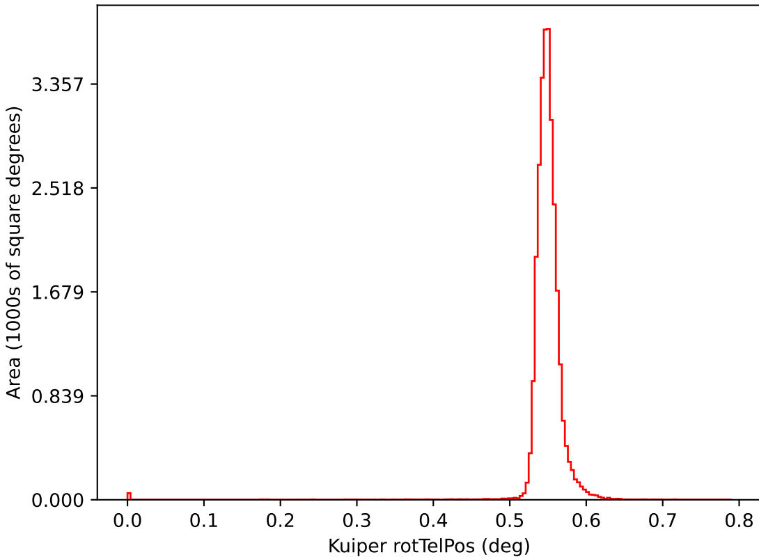
too_elab_r64_d3_giz_v3.4_10yrs i: Kuiper rotTelPos
