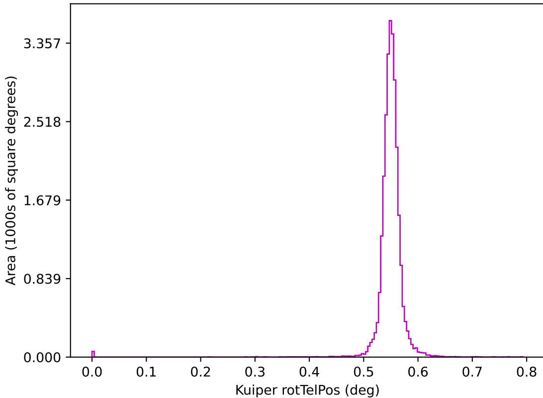
too_elab_r64_d2_ugrizy_v3.4_10yrs z: Kuiper rotTelPos
