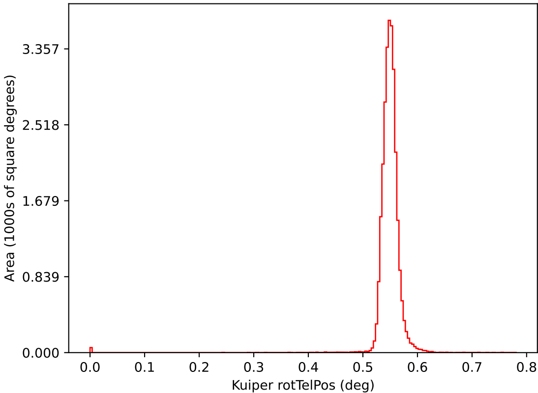
too_elab_r64_d2_ugrizy_v3.4_10yrs i: Kuiper rotTelPos
