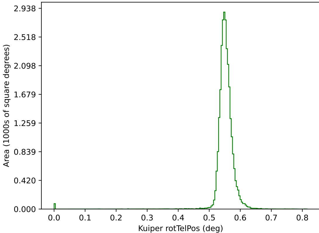
too_elab_r64_d2_ugrizy_v3.4_10yrs g: Kuiper rotTelPos
