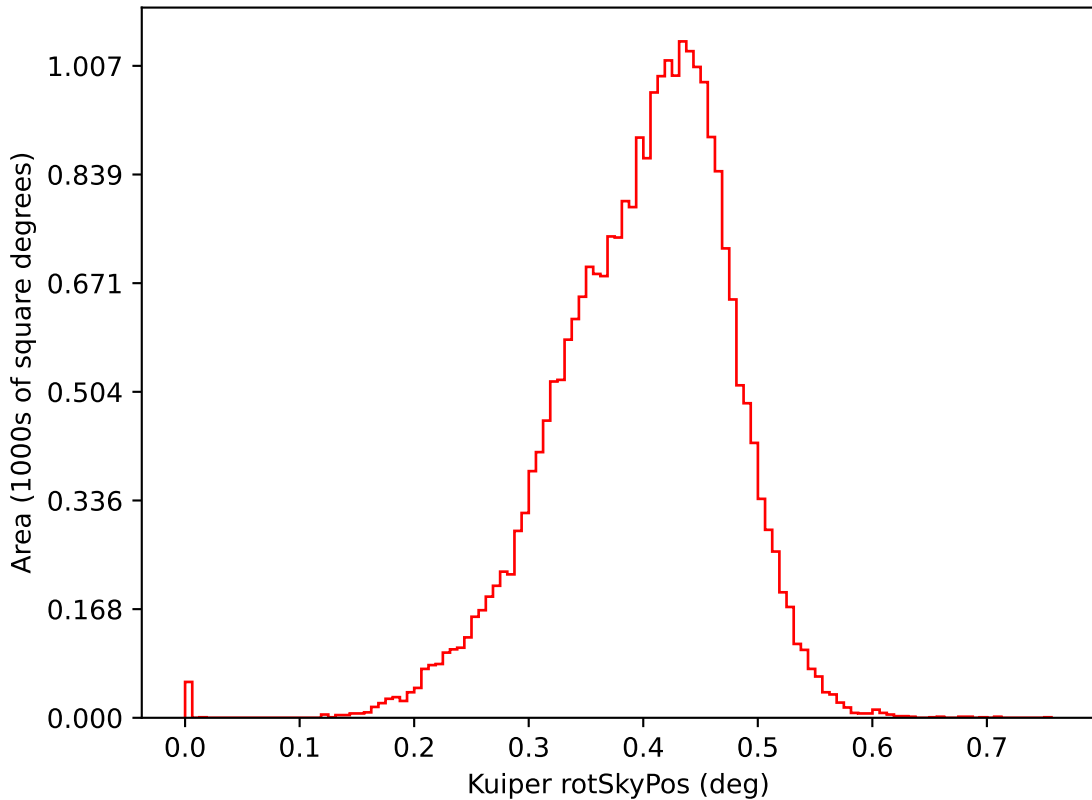
too_elab_r64_d2_ugrizy_v3.4_10yrs i: Kuiper rotSkyPos
