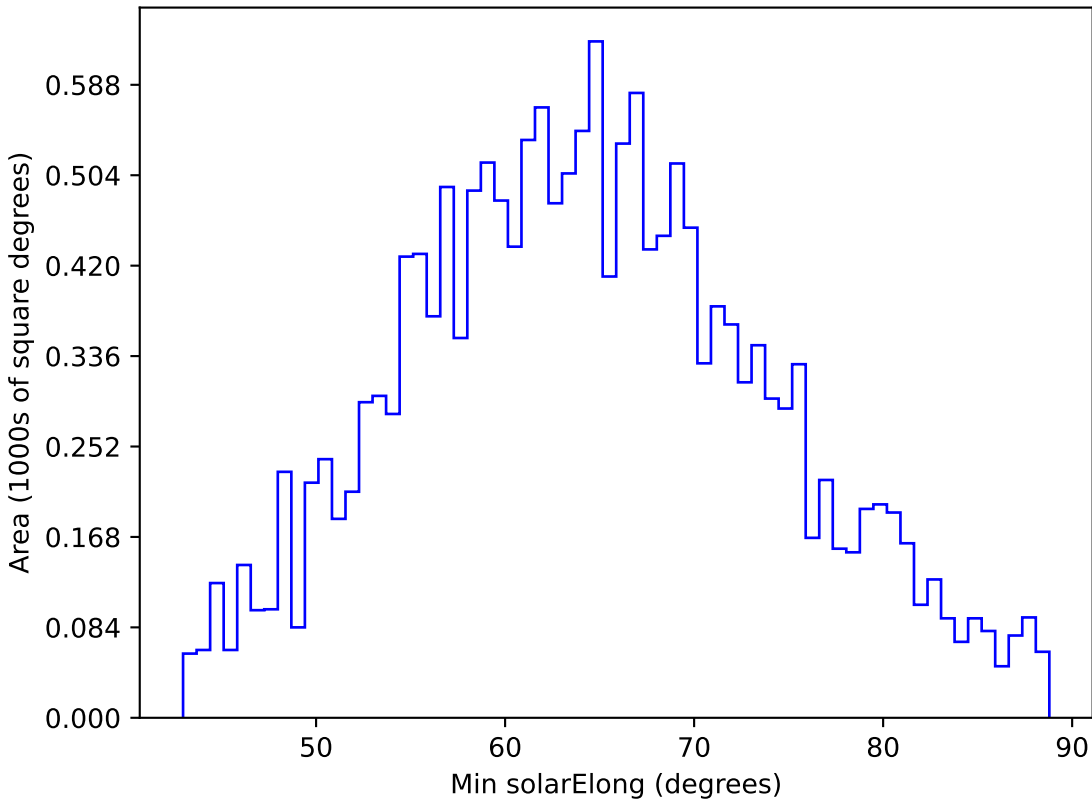
too_elab_r64_d2_ugrizy_v3.4_10yrs WFD y band: Min solarElong
