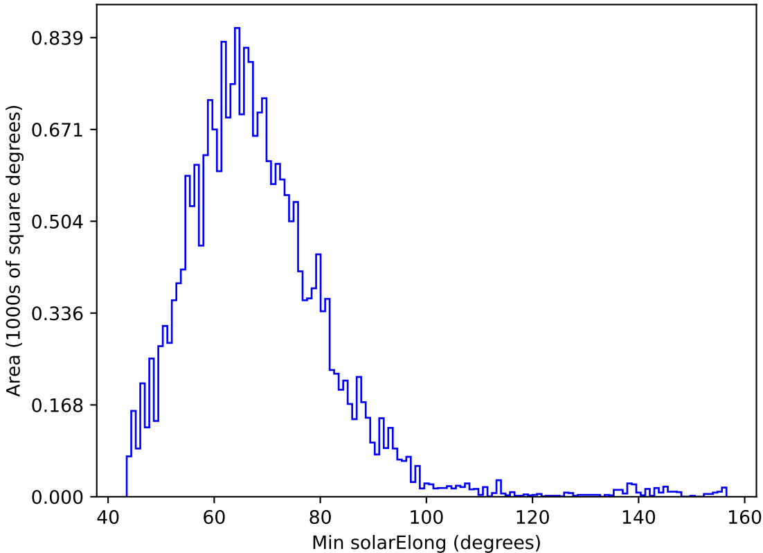
too_elab_r64_d2_ugrizy_v3.4_10yrs All sky y band: Min solarElong
