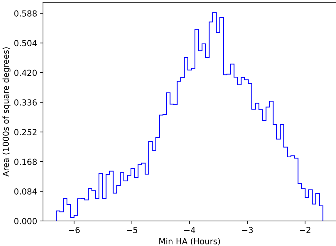
too_elab_r64_d2_ugrizy_v3.4_10yrs WFD y band: Min HA
