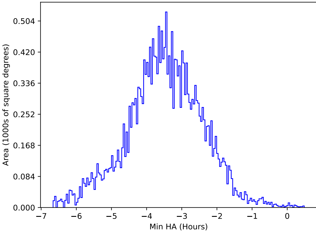
too_elab_r64_d2_ugrizy_v3.4_10yrs All sky y band: Min HA
