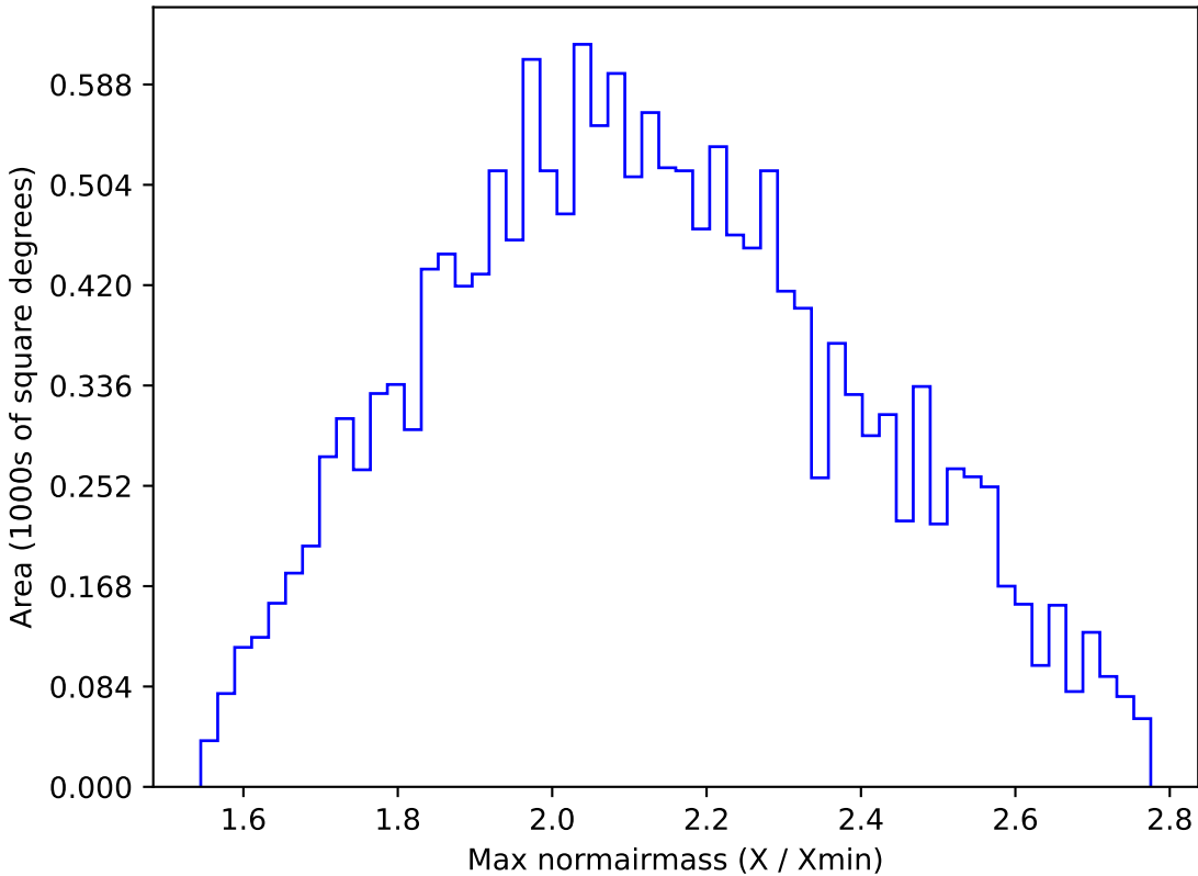
too_elab_r64_d2_ugrizy_v3.4_10yrs WFD y band: Max normairmass
