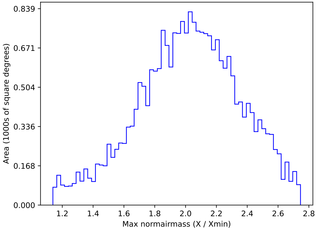
too_elab_r64_d2_ugrizy_v3.4_10yrs All sky y band: Max normairmass
