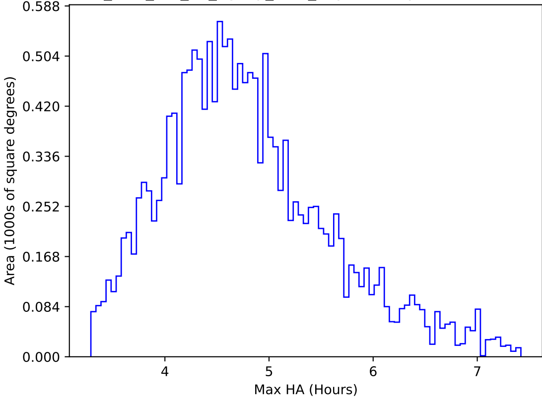
too_elab_r64_d2_ugrizy_v3.4_10yrs WFD y band: Max HA
