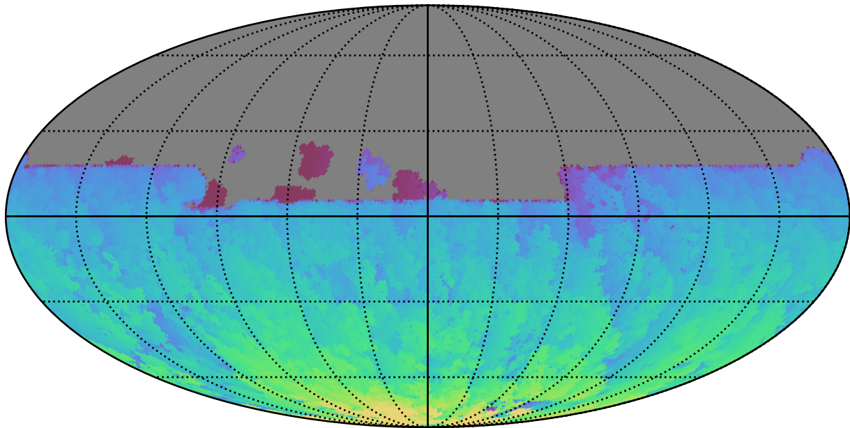
too_elab_r64_d2_ugrizy_v3.4_10yrs All sky y band: Max HA
