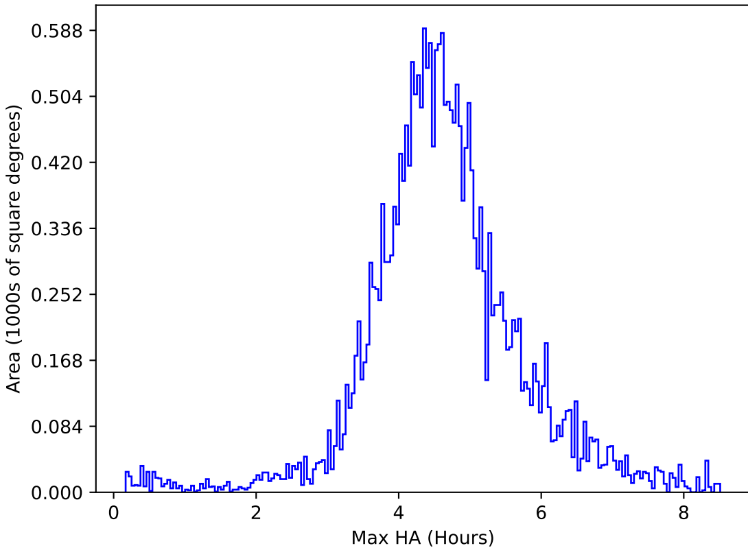
too_elab_r64_d2_ugrizy_v3.4_10yrs All sky y band: Max HA
