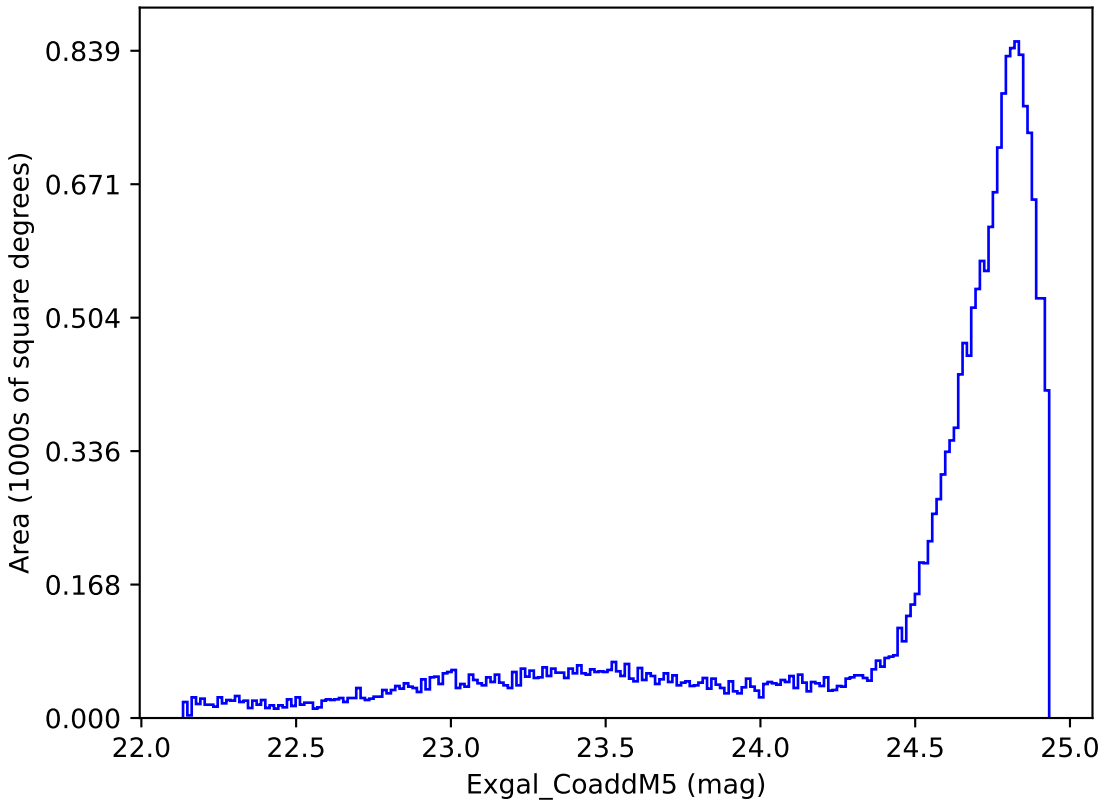
too_elab_r64_d2_ugrizy_v3.4_10yrs All sky y band: Exgal_CoaddM5
