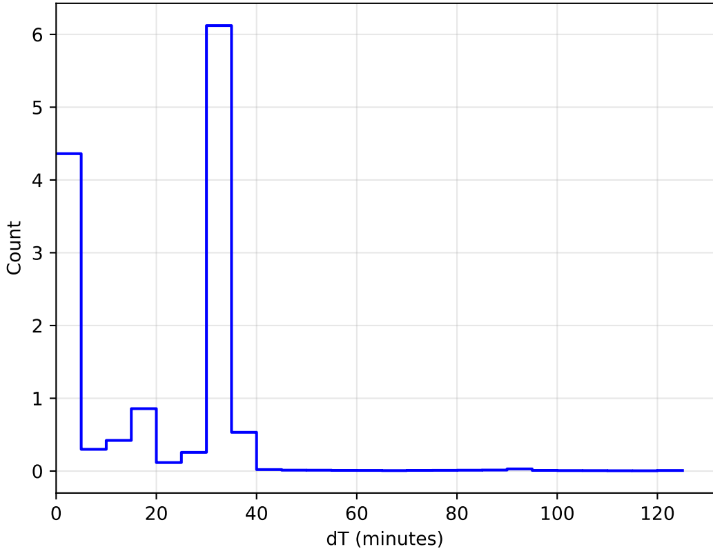
too_elab_r64_d2_ugrizy_v3.4_10yrs All sky: DeltaT Histogram 1e6
