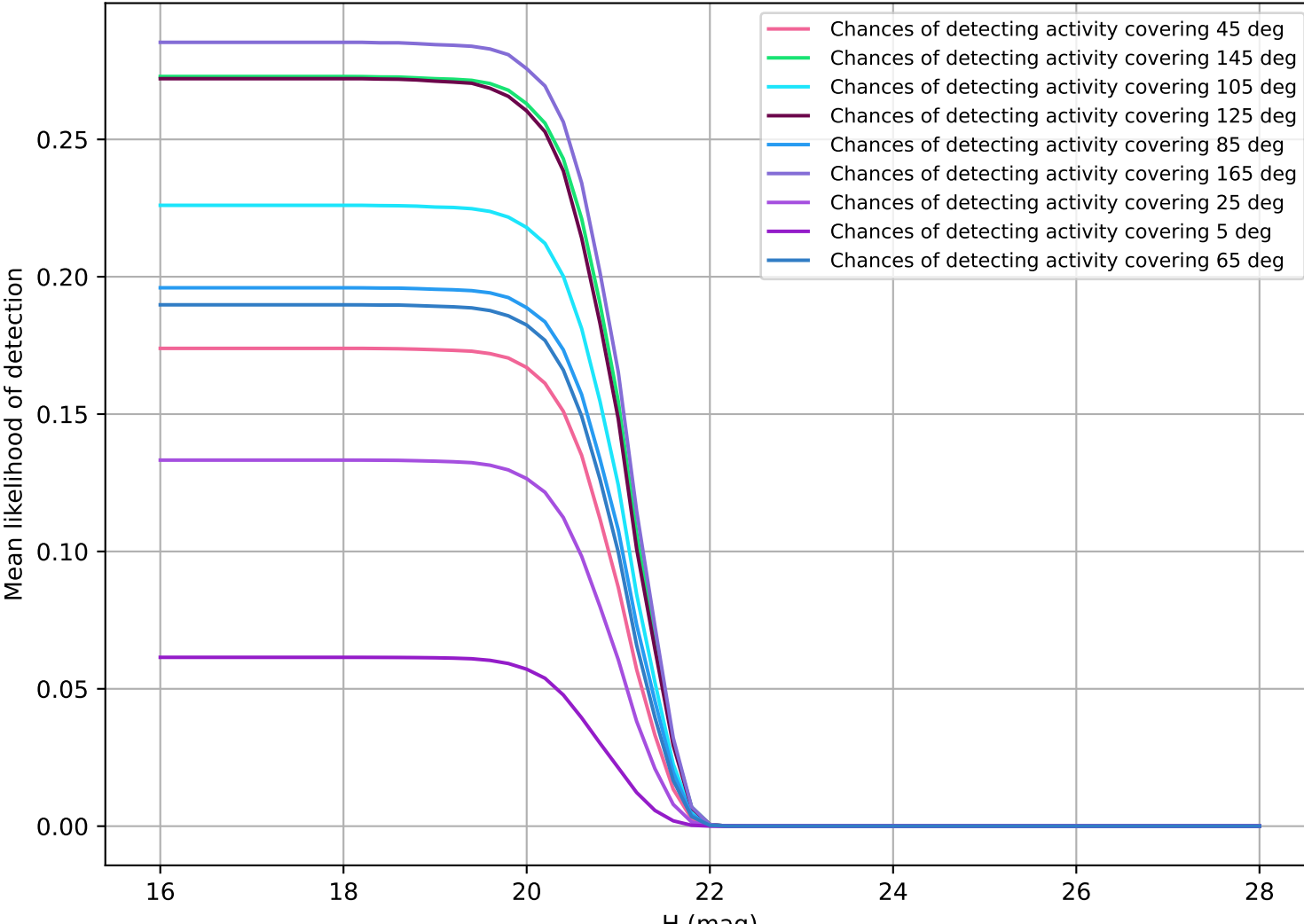
too elab r64 d2 gz v3.4 10yrs Vatira
