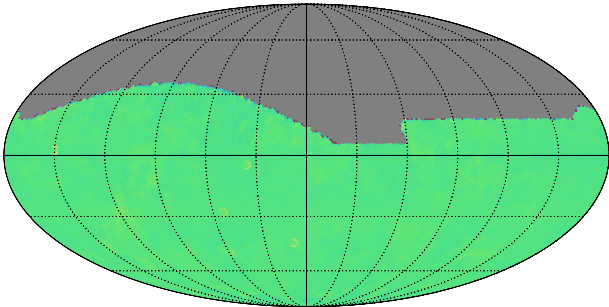
too_elab_r64_d2_gz_v3.4_10yrs i: Kuiper rotTelPos
