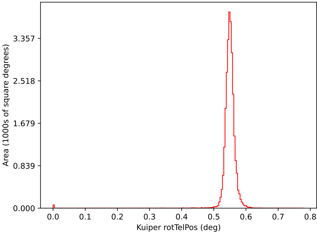
too_elab_r64_d2_gz_v3.4_10yrs i: Kuiper rotTelPos
