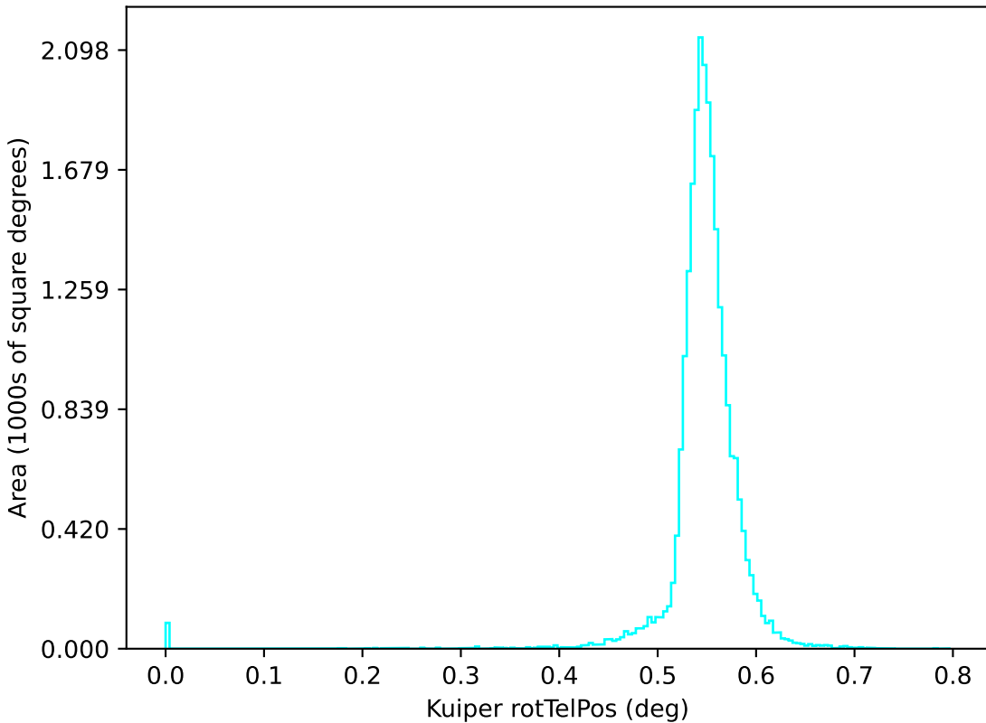
too_elab_r64_d2_griz_v3.4_10yrs u: Kuiper rotTelPos
