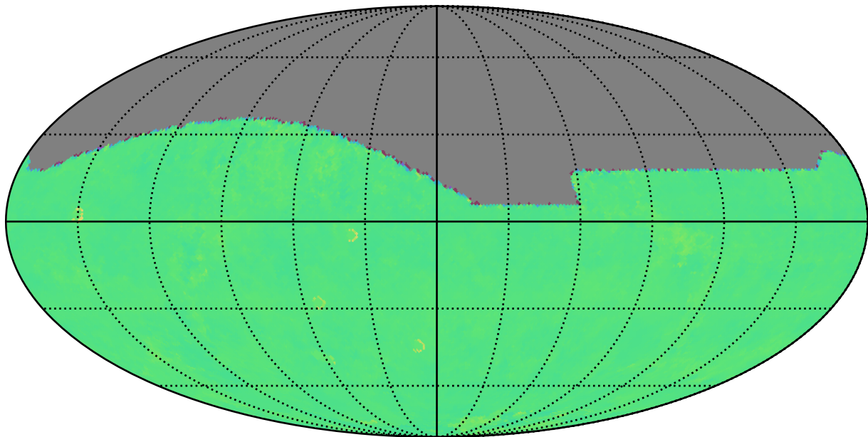
too_elab_r64_d2_griz_v3.4_10yrs i: Kuiper rotTelPos
