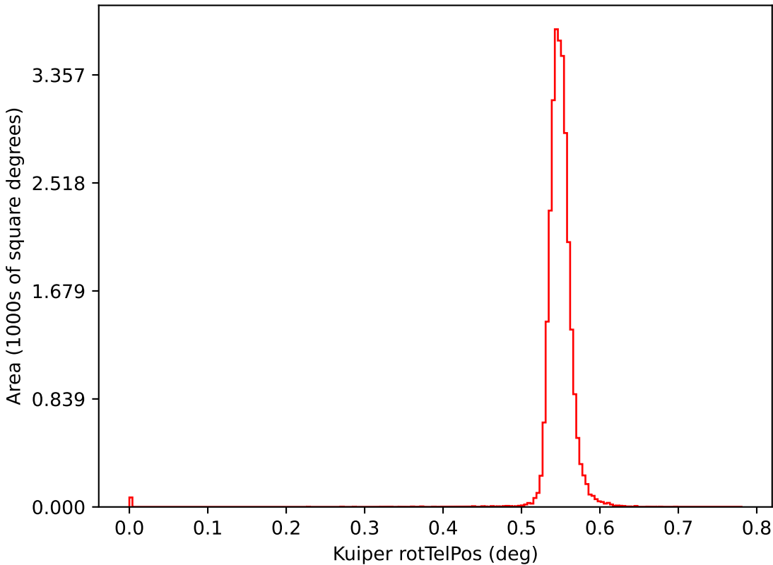
too_elab_r64_d2_griz_v3.4_10yrs i: Kuiper rotTelPos
