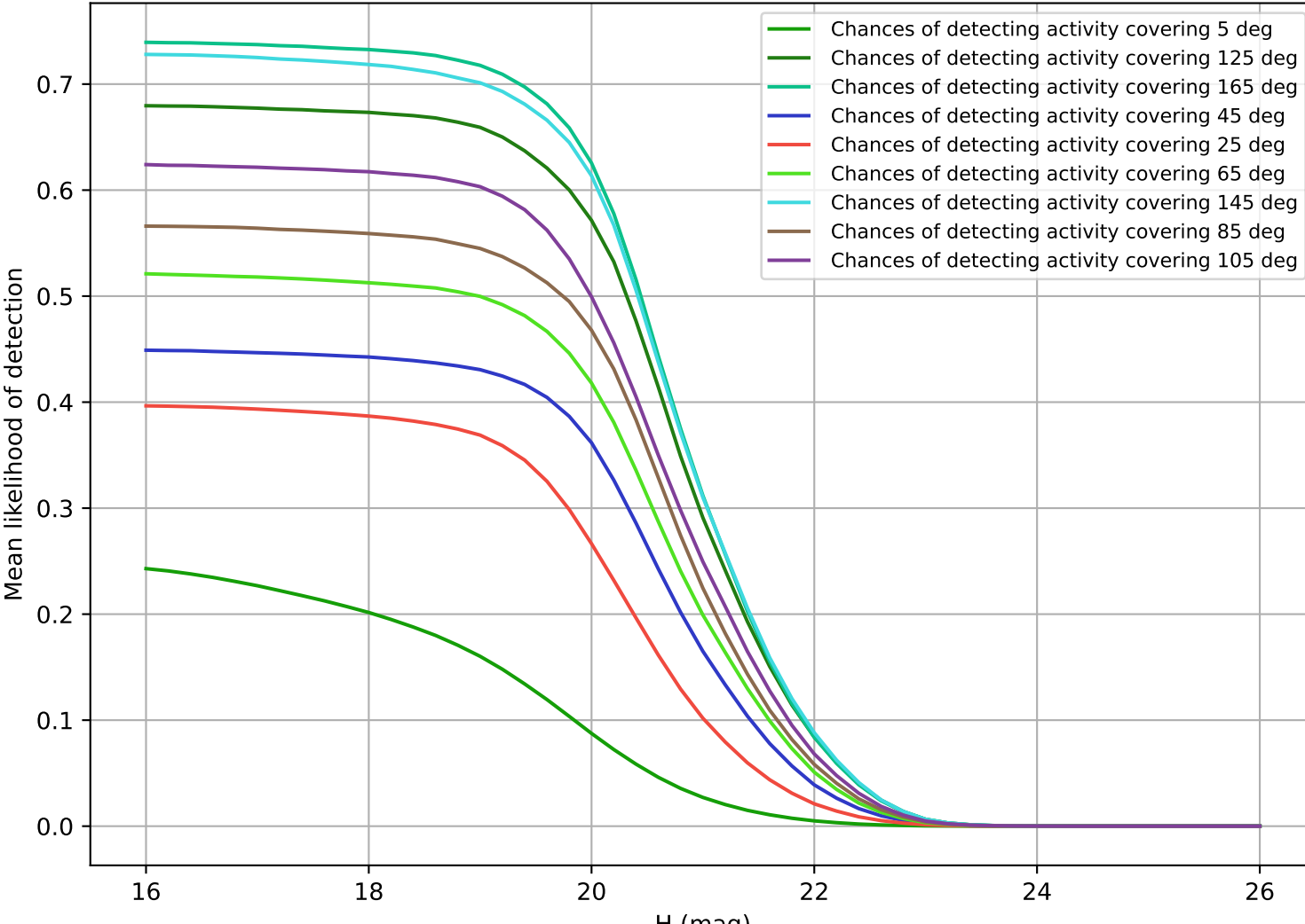
too elab r64 d2 giz v3.4 10yrs MBA
