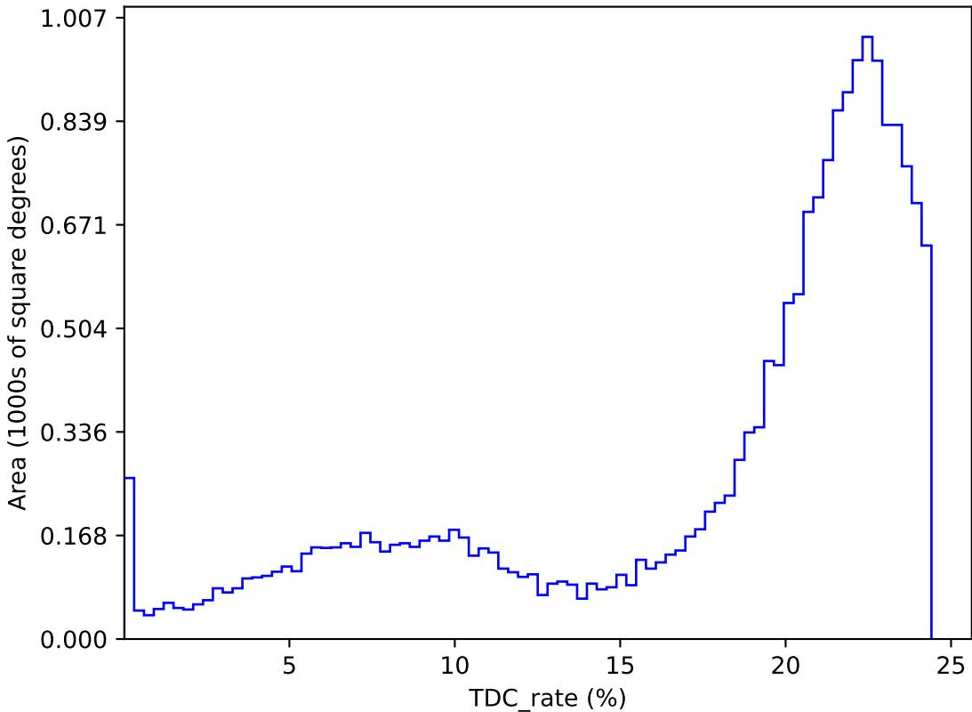
too_elab_r32_d3_ugrizy_v3.4_10yrs : TDC_rate
