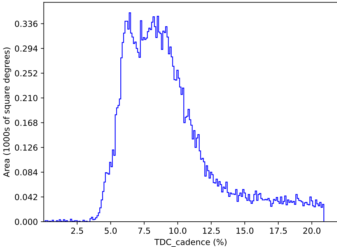
too_elab_r32_d3_ugrizy_v3.4_10yrs : TDC_cadence
