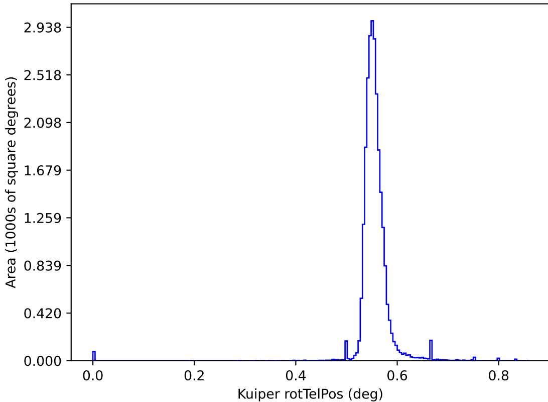
too_elab_r32_d3_ugrizy_v3.4_10yrs y: Kuiper rotTelPos
