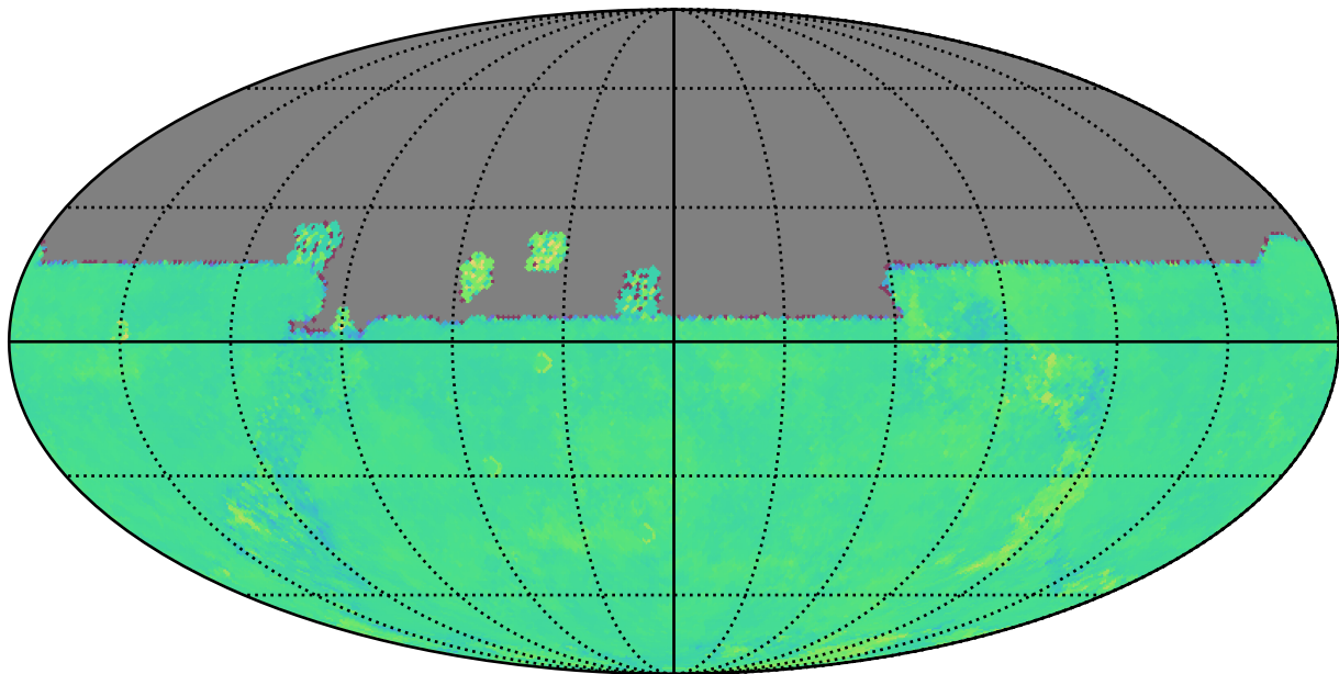
too_elab_r32_d3_ugrizy_v3.4_10yrs u: Kuiper rotTelPos
