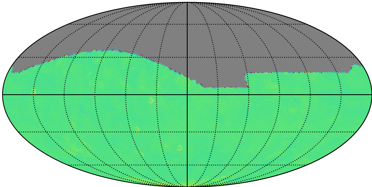
too_elab_r32_d3_ugrizy_v3.4_10yrs r: Kuiper rotTelPos
