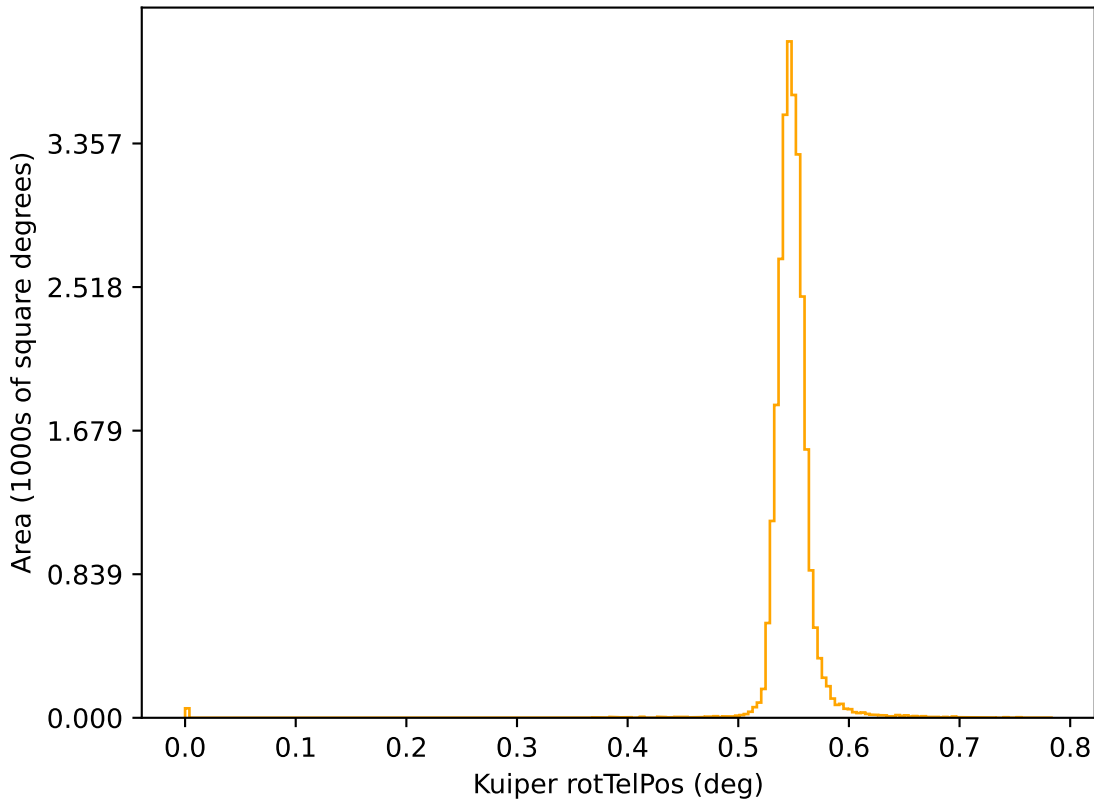
too_elab_r32_d3_ugrizy_v3.4_10yrs r: Kuiper rotTelPos
