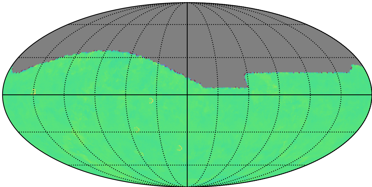
too_elab_r32_d3_ugrizy_v3.4_10yrs i: Kuiper rotTelPos
