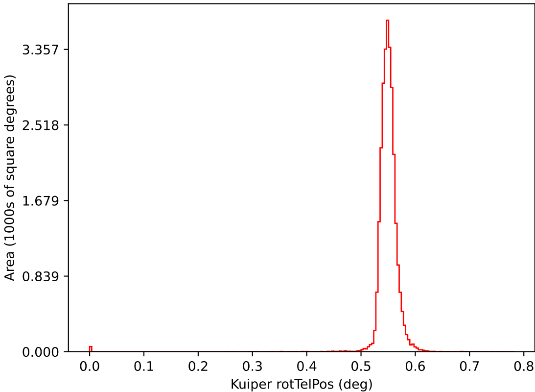
too_elab_r32_d3_ugrizy_v3.4_10yrs i: Kuiper rotTelPos
