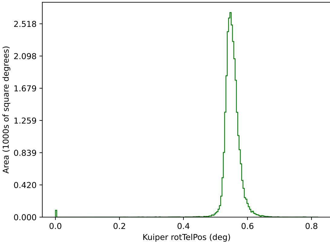
too_elab_r32_d3_ugrizy_v3.4_10yrs g: Kuiper rotTelPos
