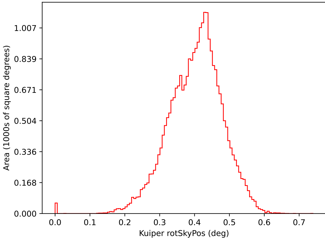
too_elab_r32_d3_ugrizy_v3.4_10yrs i: Kuiper rotSkyPos
