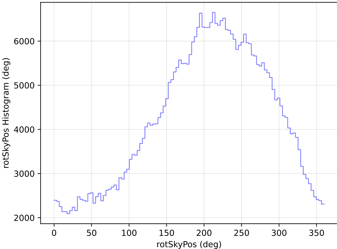
too_elab_r32_d3_ugrizy_v3.4_10yrs WFD z band: rotSkyPos Histogram
