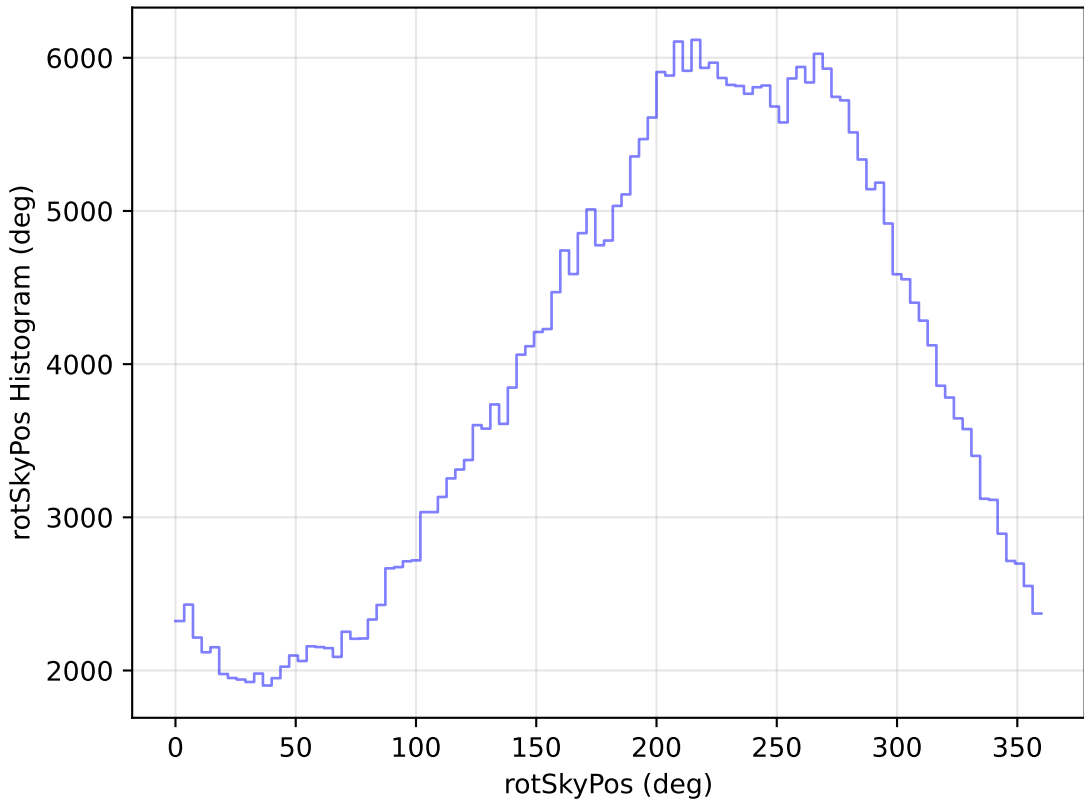
too_elab_r32_d3_ugrizy_v3.4_10yrs WFD y band: rotSkyPos Histogram
